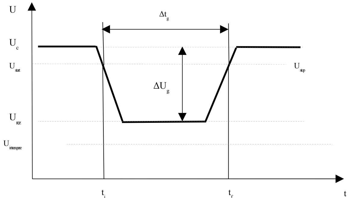
Fig. 1: Forma simplificată a unui gol de tensiune
